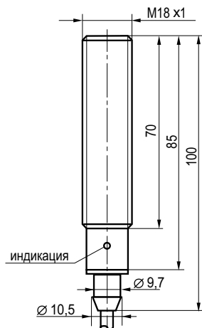
Габаритный чертеж
